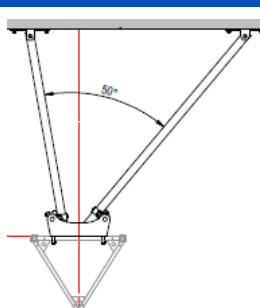
ANCLAJE
