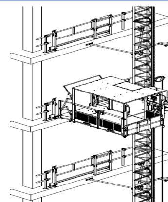
VISTA LATERAL
