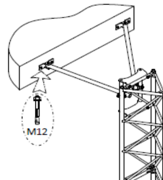
VISTA ARRIOSTRAMIENTO
